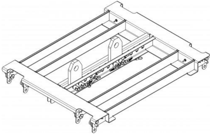
E 系列悬挂框架
